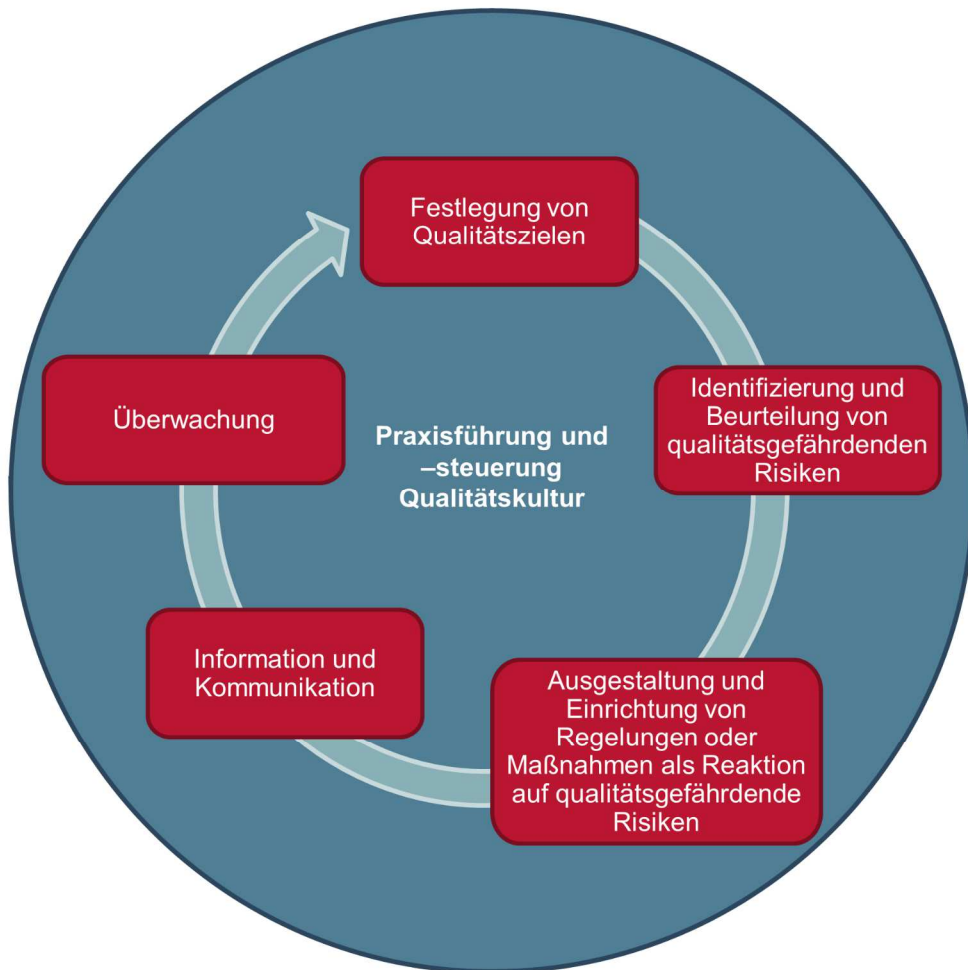
Abb.: Qualitätsmanagement-Prozess
